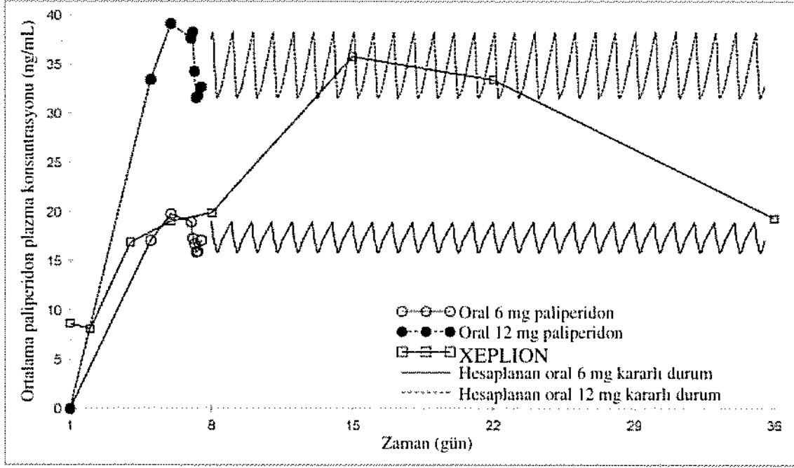
Şekil 2. Oral uzatılmış salımlı tabletin (6 mg veya 12 mg) günlük uygulaması ile karşılaştırılabilir olarak önerilen başlangıç rejimi kullanılarak (1.gün/8.günde deltoid kas içine 150 mg/100 mg paliperidona eşdeğer paliperidon palmitat ile başlangıç) XEPLION'un uygulamasını takiben 5 hafta süre ile paliperidon için ortalama farmakokinetik profillerini takiben ortalama plazma konsantrasyonu-zaman profilleri.
